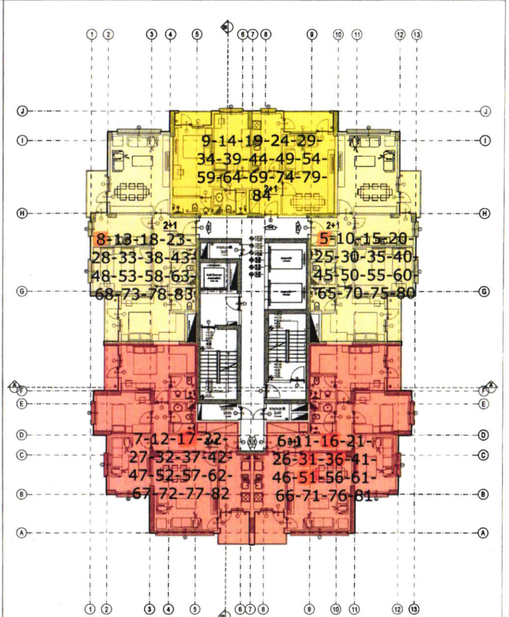
B1 BLOK +3.00,+6.00,+9.00,+12.00,+15.00,+18.00 Kotları 1,2,3,4,5,6. NORMAL KAT PLANI ÖLÇEK: 1/100 Alan= 604,70 m 2
