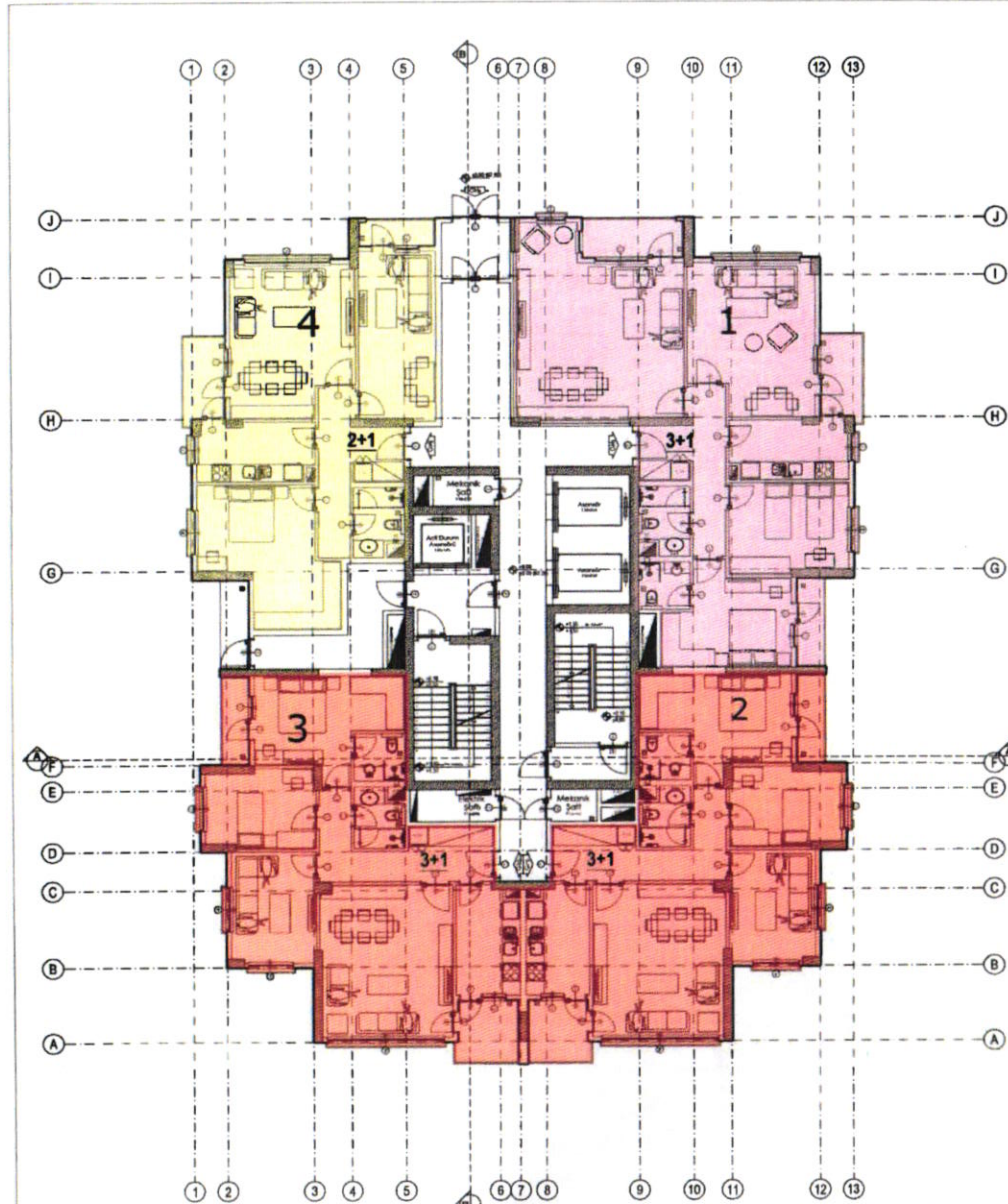
B1 BLOK ±0,00(67,00) Kotu ZEMİN KAT PLANI ÖLÇEK: 1/100 Alan= 604,70 m 2
